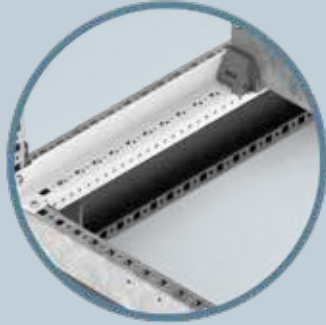
Montaj kolaylığı sağlayan kızaklı ve tekerlekli montaj plakası tasarımı.
