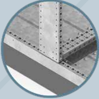
Yatay ve dikey bölme takımındaki özel tespit sayesinde birleşim noktasındaki sızdırmalık arttırılmıştır.
