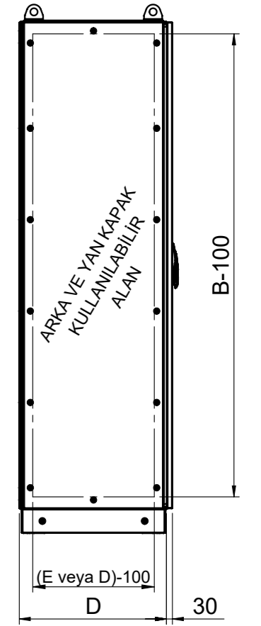
YAN GÖRÜNÜŞ
