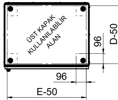
ÜST GÖRÜNÜŞ
