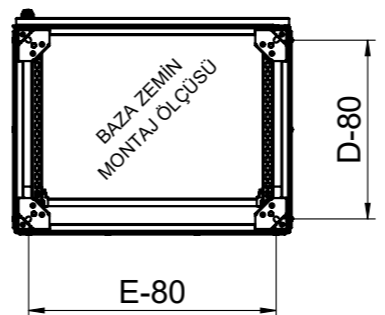
ALT GÖRÜNÜŞ
