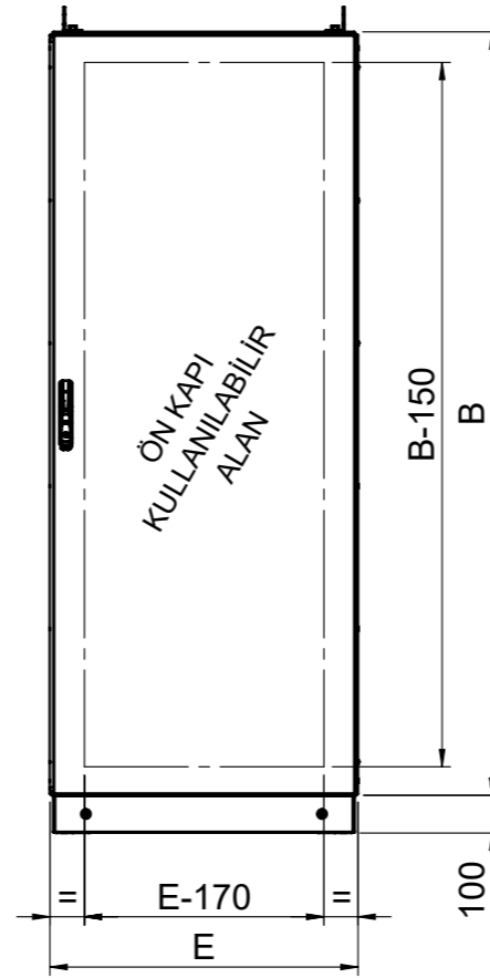
ÖN GÖRÜNÜŞ
